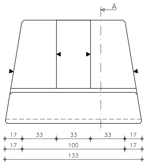
BOVENZIJDE
