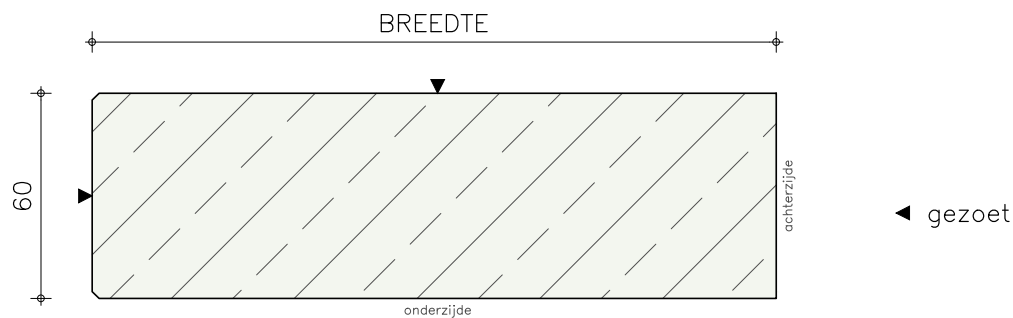
Standaard zijaanzicht/doorsnede
