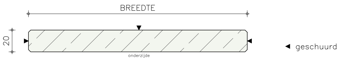
Standaard zijaanzicht/doorsnede
