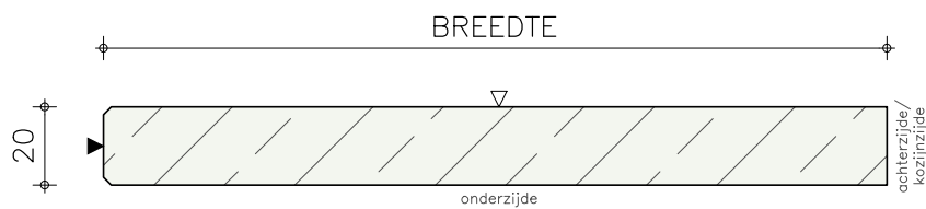
Standaard zijaanzicht/doorsnede
