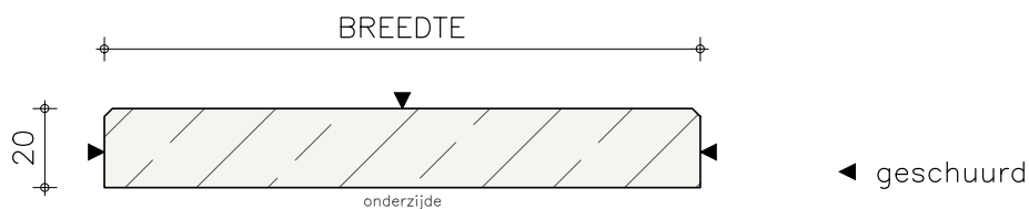
Standaard zijaanzicht/doorsnede
