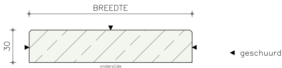
Standaard zijaanzicht/doorsnede
