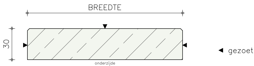
Standaard zijaanzicht/doorsnede
