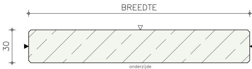
Standaard zijaanzicht/doorsnede
