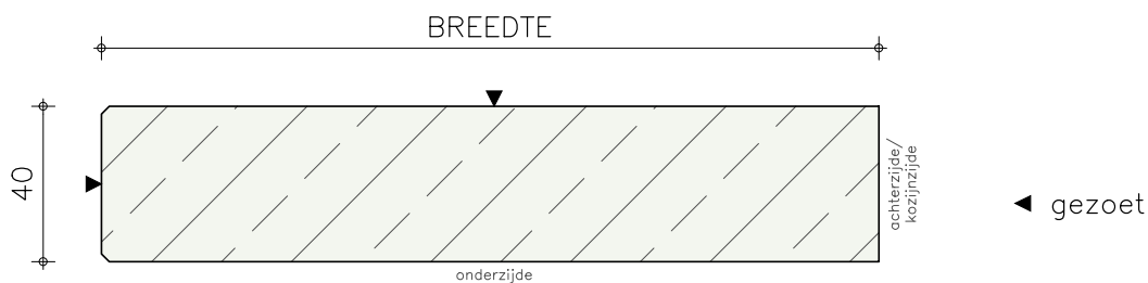
Standaard zijaanzicht/doorsnede
