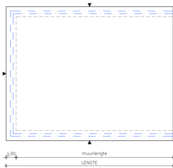
BOVENAANZICHT
