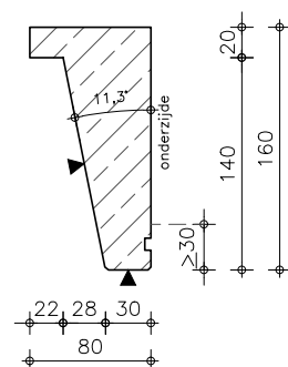
ZIJAAANZ./DRSN.
