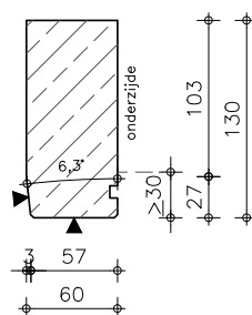
ZIJAAANZ./DRSN.
